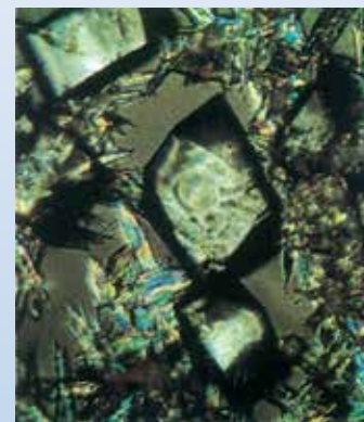
Kristali karbonatov obdelani s Polarjem, so sprijeti in potujejo naprej skupaj z vodo z manj nalaganja na cevi in površine.
